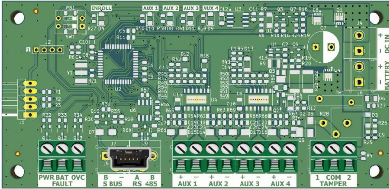
PS-5U
