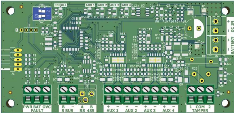
PS-55B
